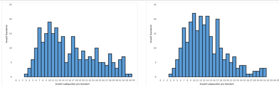
Abbildung 15: Anzahl Ladepunkte ohne (links) und mit (rechts) 2.000 km Basisnetz Oberleitung
