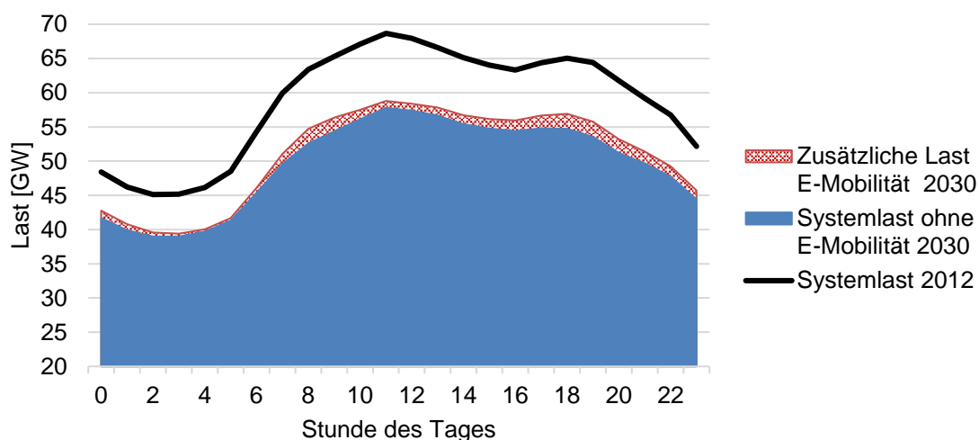
Abbildung 5: Mittlere Systemlast Deutschlands für die Jahre 2012 (Linie) und 2030 (Fläche). Für das Jahr 2030 zeigt die rote Fläche die Last privater Elektrofahrzeuge (3,7 kW-Szenario).
