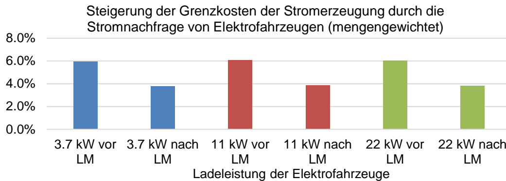
Abbildung 8: Ermittlung der prozentualen Zunahme der Grenzkosten der Stromerzeugung unter Berücksichtigung von Ladeleistung und Lastmanagement (LM)
