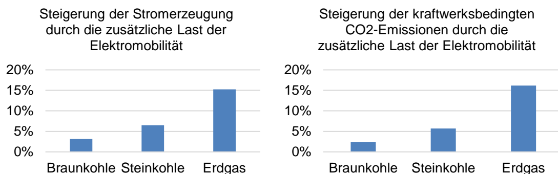
Abbildung 9: Auswirkungen der Diffusion der Elektromobilität und der damit einhergehenden zusätzlichen Stromnachfrage auf die Stromerzeugung. Vergleich der Stromerzeugung exkl. privater Elektrofahrzeuge mit dem Szenario 3,7 kW ohne Lastmanagement
