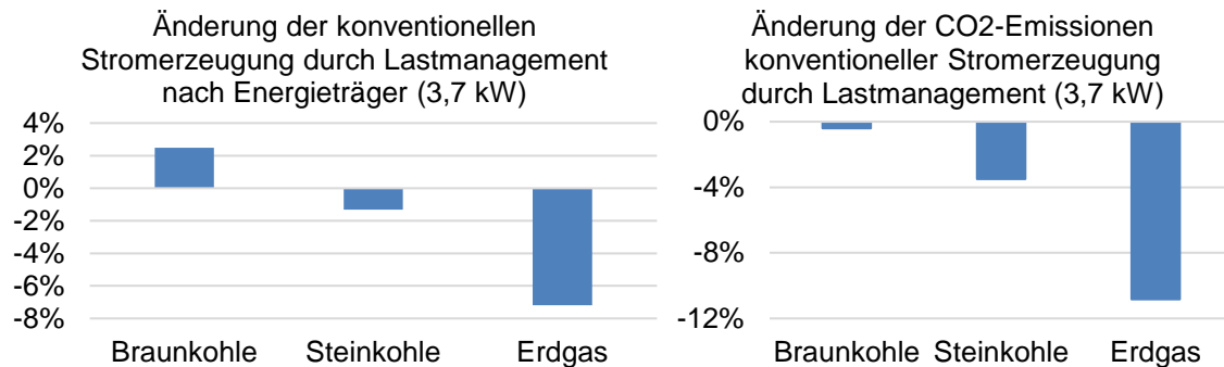
Abbildung 10: Auswirkungen von Lastmanagement auf den Einsatz konventioneller Kraftwerke sowie die kraftwerksbedingten CO 2 -Emissionen im Szenario 3,7 kW
