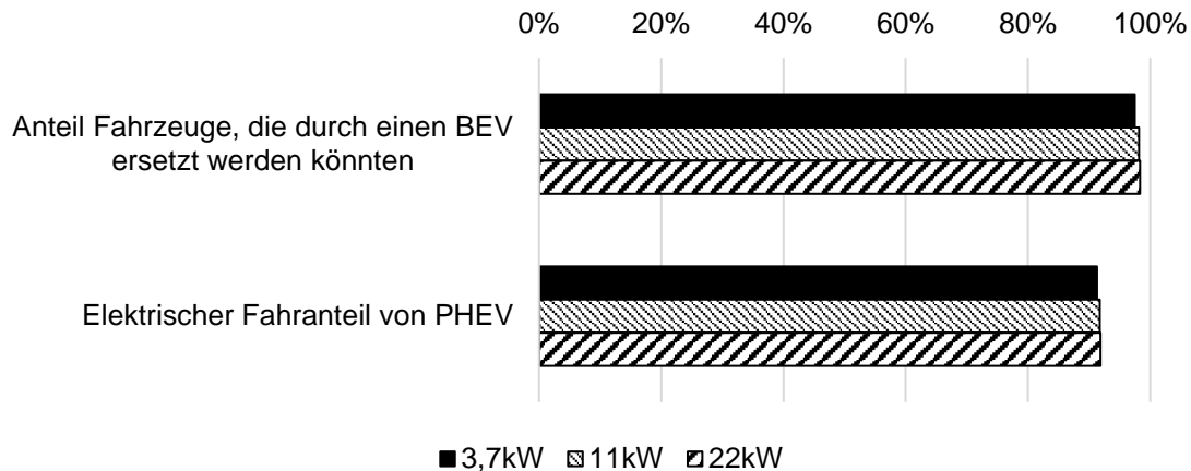
Abbildung 4: Einfluss der Ladeleistung auf den Einsatz von BEV und PHEV aus technischer Sicht mit Annahmen für 2030
