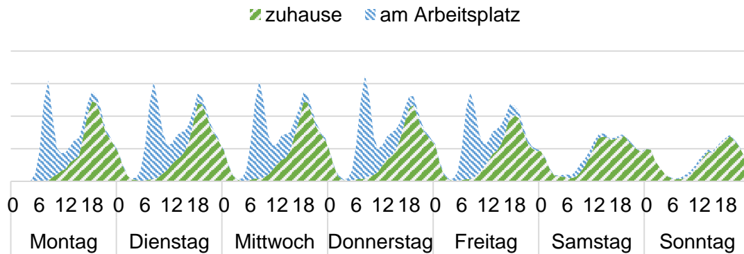
Abbildung 3: Simulierter Lastverlauf von privaten Elektrofahrzeugen, wenn Lademöglichkeiten zu Hause und am Arbeitsplatz bestehen (hier 3,7 kW)
