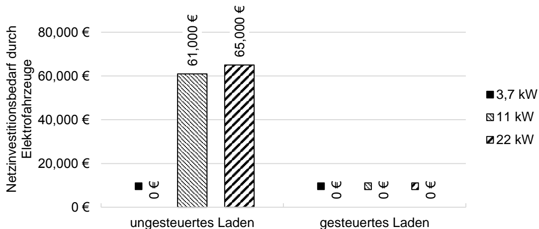
Abbildung 13: Investitionsbedarf für das Netz aus Abbildung 12 in Abhängigkeit der Elektrofahrzeugdurchdringung und der Ladeleistung der Fahrzeuge
