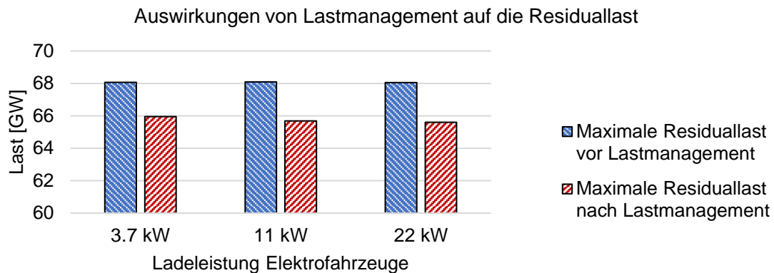
Abbildung 7: Maximale Residuallast vor und nach dem Lastmanagementsinsatz von Elektrofahrzeugen unter Berücksichtigung der Ladeleistung
