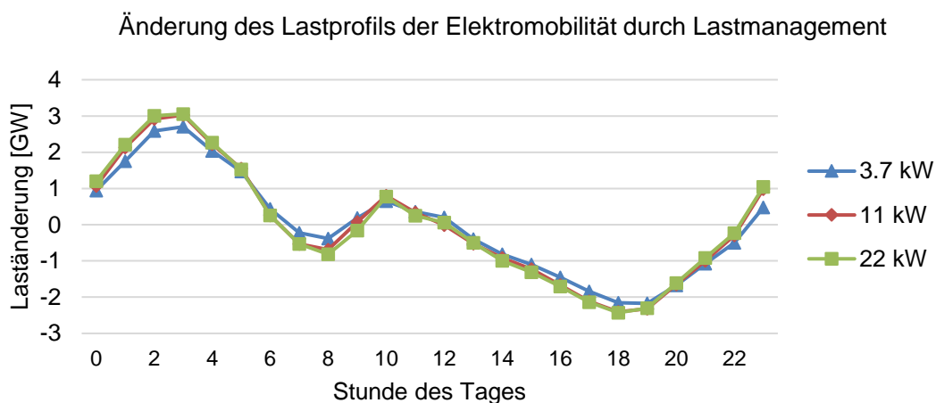
Abbildung 6: Laständerung von privaten Elektrofahrzeugen nach Lastmanagementoptimierung unter Berücksichtigung der Ladeleistung
