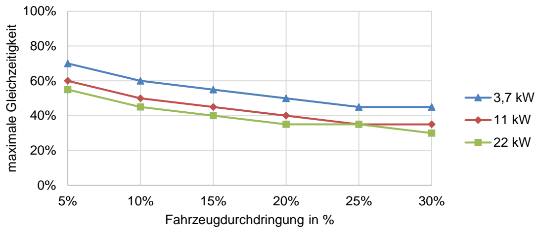
Abbildung 11: Maximale Gleichzeitigkeit für verschiedene Ladeleistungen und Elektrofahrzeugdurchdringungen [48, 49]
