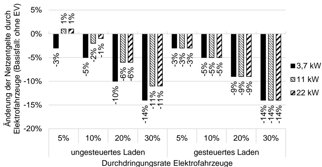
Abbildung 14: Einfluss der zusätzlichen Stromnachfrage durch Elektrofahrzeuge auf Netzentgelte in einem vorstädtischen Netz
