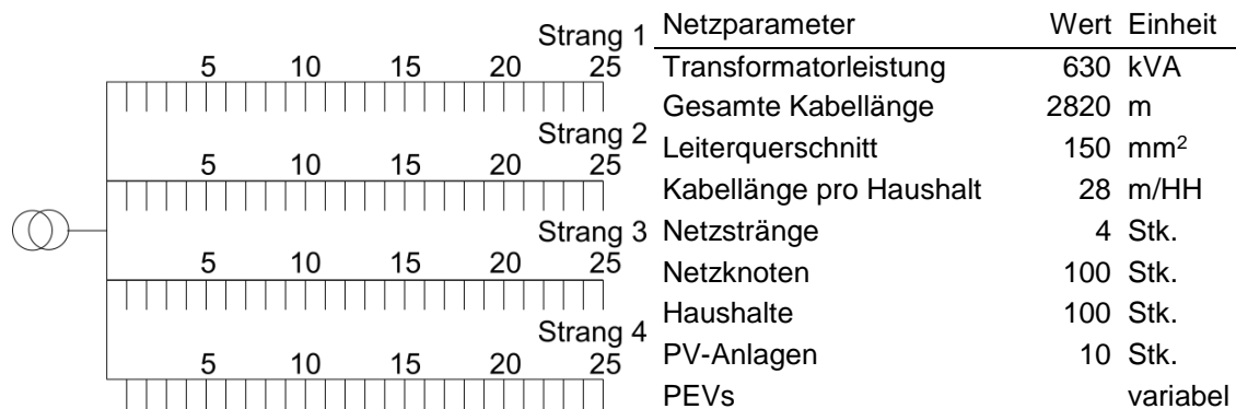
Abbildung 12: Topologie des vorstädtischen Netzes sowie die verwendeten Netzparameter
