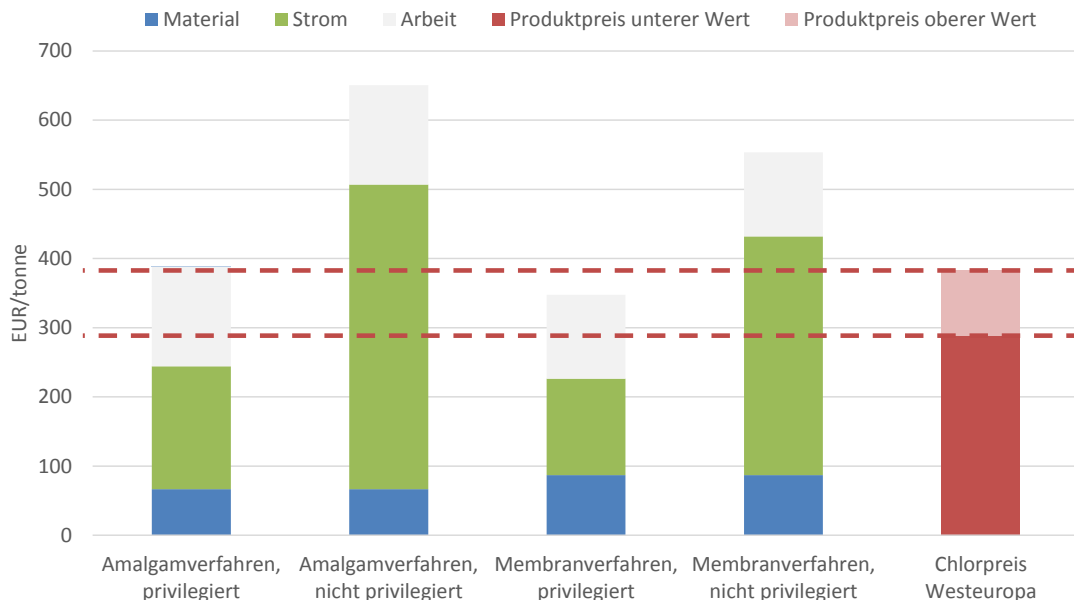
Abbildung 21: Bestandteile der Produktionskosten in der Chlorproduktion
